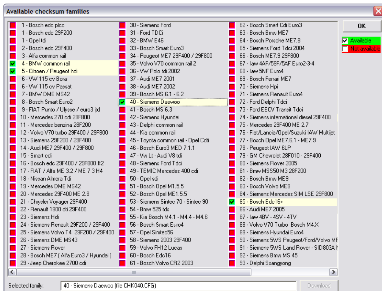
Figure 13: fenêtre des familles de Somme de Contrôle disponibles mise à jour.
